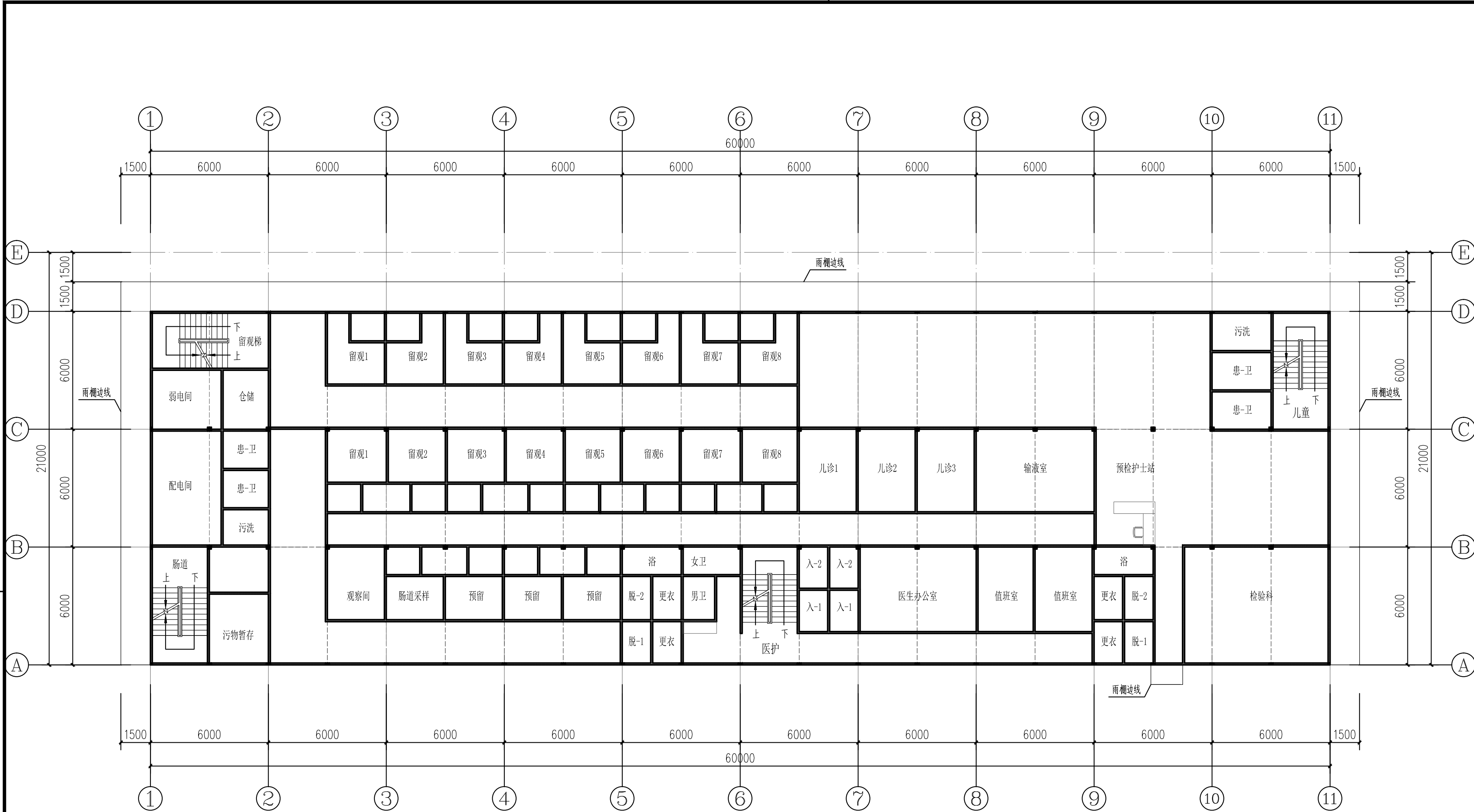
二层平面图 1:150 本层建筑面积：1080平方米 二层：儿童普通发热门诊 成人普通发热门诊 隔离留观室
