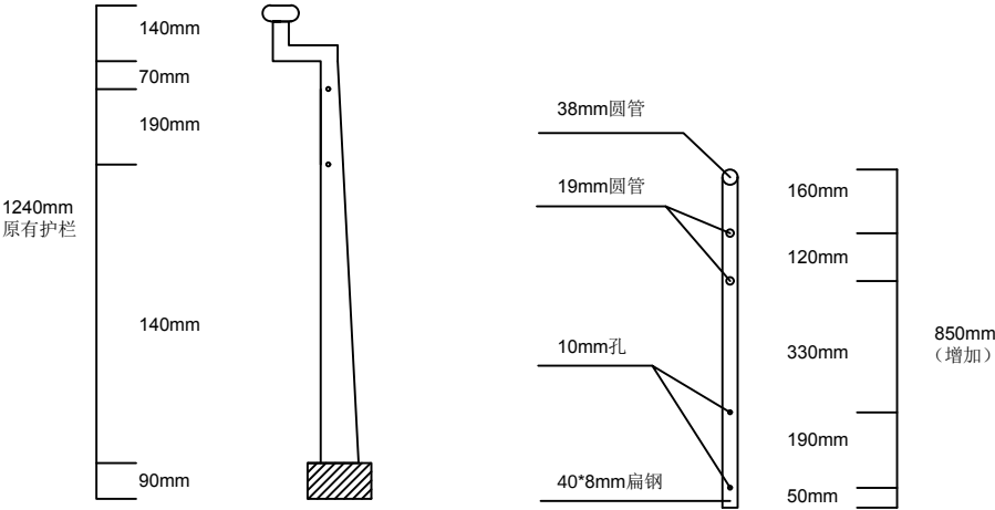
门诊二，三，四楼外围护栏增高示意图
